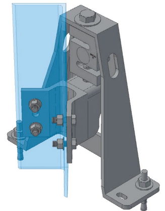
ADAPTADOR PARA PIE DE HIERRO EN ÁNGULO
