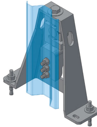
ADAPTADOR DE PIE ESTÁNDAR
