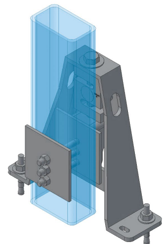
ADAPTADOR PARA PIE EN FORMA DE TUBO
