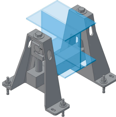
ADAPTADOR PARA VIGAS EN DOBLE T
